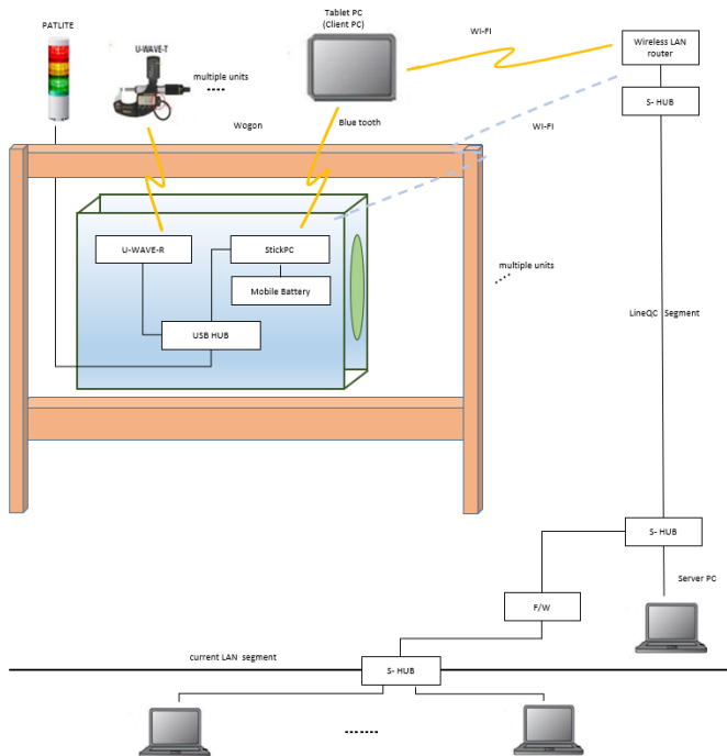
システム構成例 クライアントサーバタイプ
